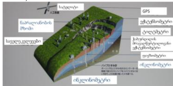
სურ. 16. მეწყერულ პროცესებზე სხვადასხვა ტიპის დაკვირვება-მონიტორინგის სისტემა
