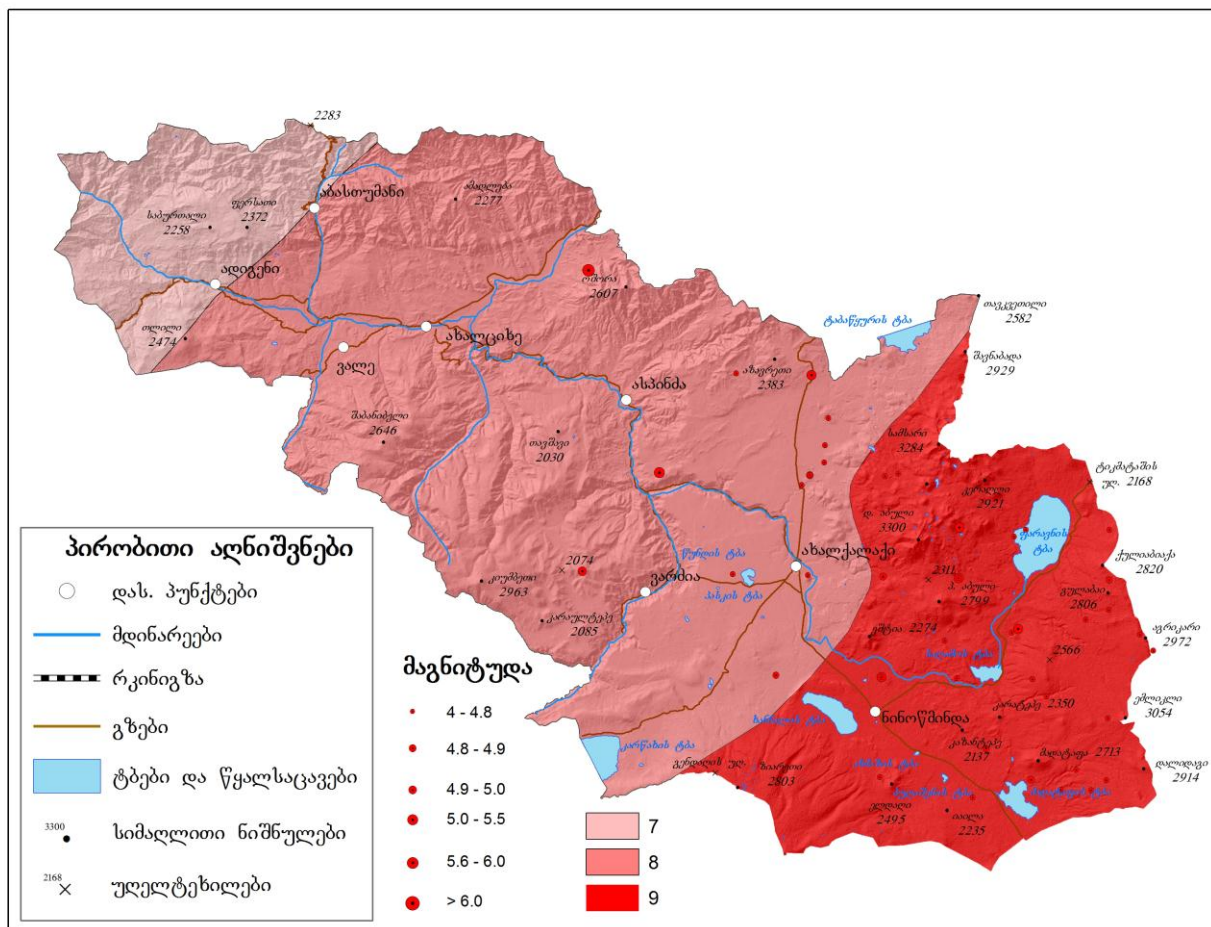
რუკა 6. საკვლევ ტერიტორიის სეისმური დარაიონება და დაფიქსირებული მიწძვრები
